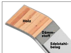
Detail Schalldämmung
